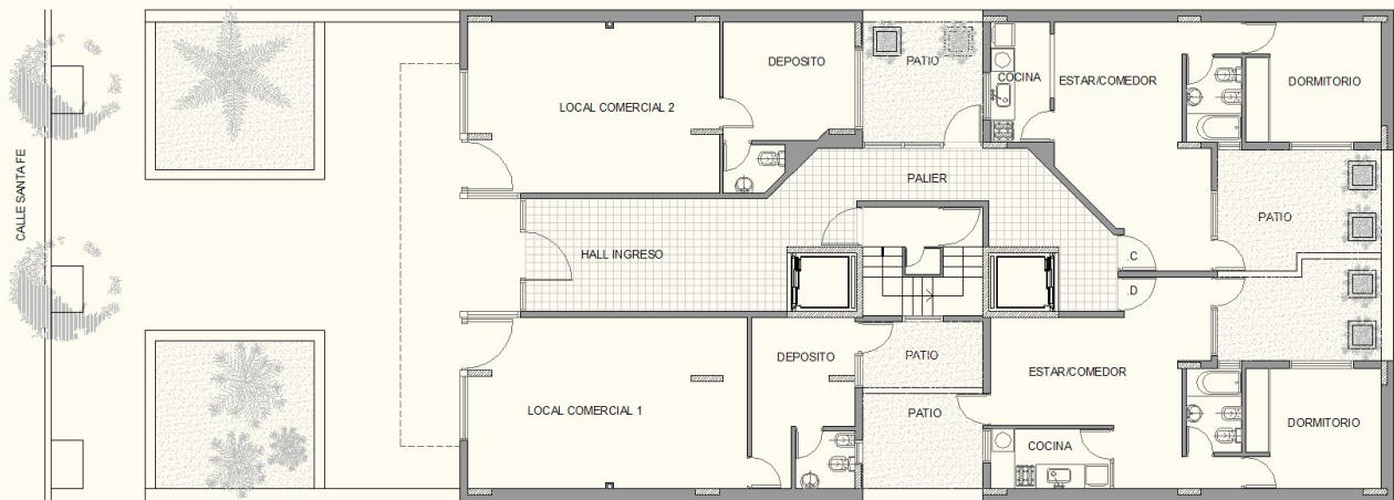
PLANTA BAJA
